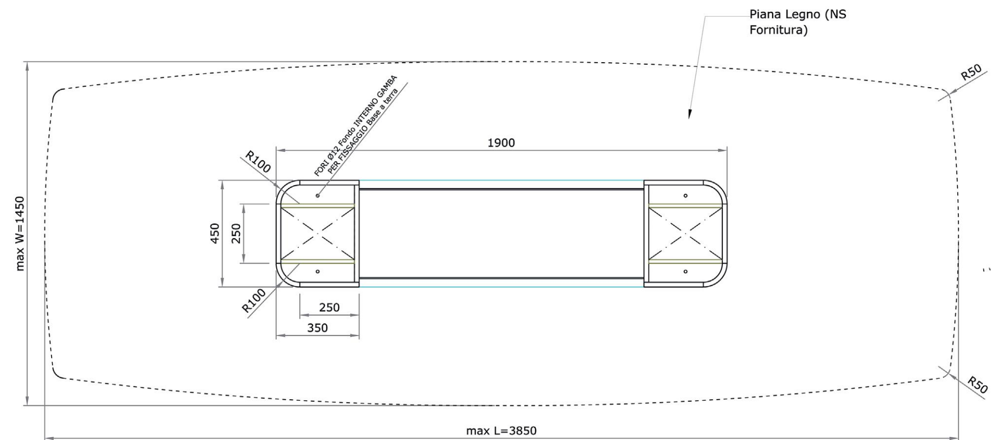
PIANTA
