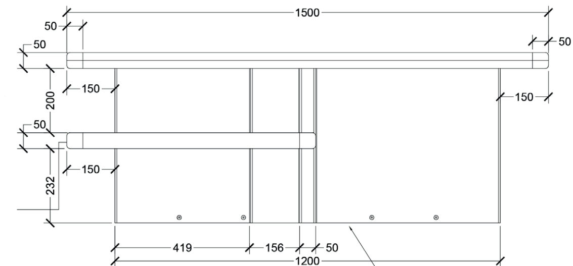
Sezione MD-A-Side Table
