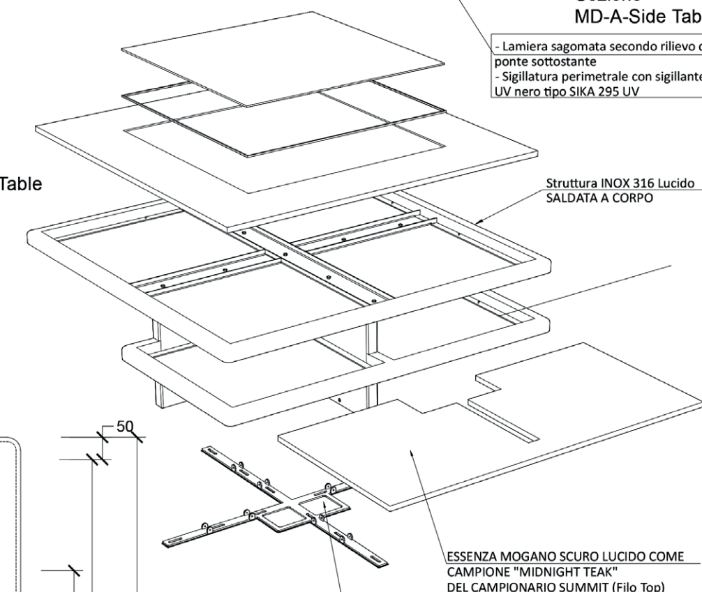
Sezione MD-A-Side Table
