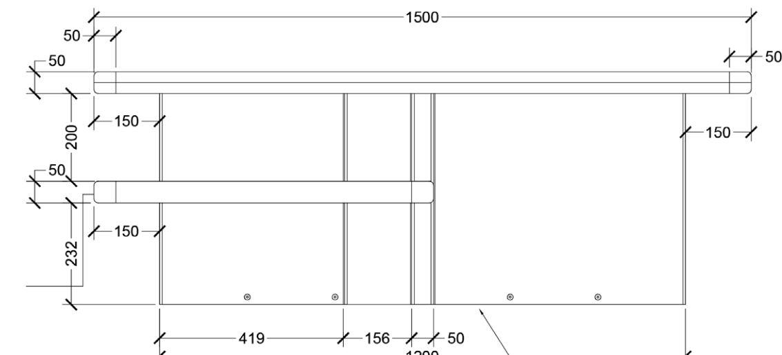
Sezione MD-A-Side Table
